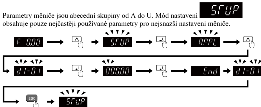
Obrázek 6.5 Parametry v módu nastavení pro univerzální účely
