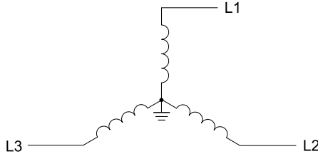
Şekil 9.8 Simetrik Topraklama
