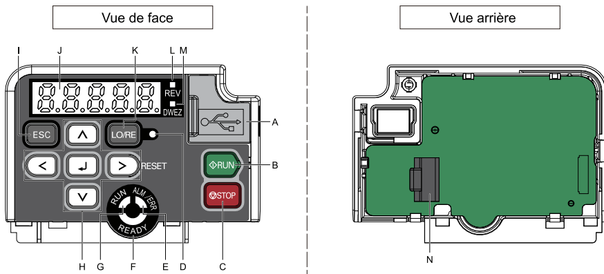
Figure 3.1 Console numérique
