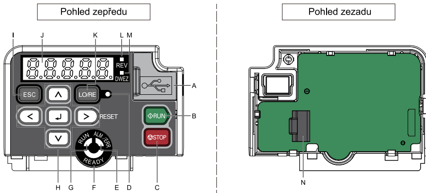
Obrázek 6.1 Klávesnice
