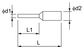
Figure 3.4 Dimensions extérieures des emboutis à sertir
