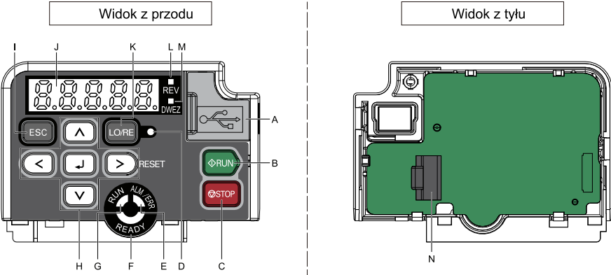
Rysunek 7.1 Klawiatura
