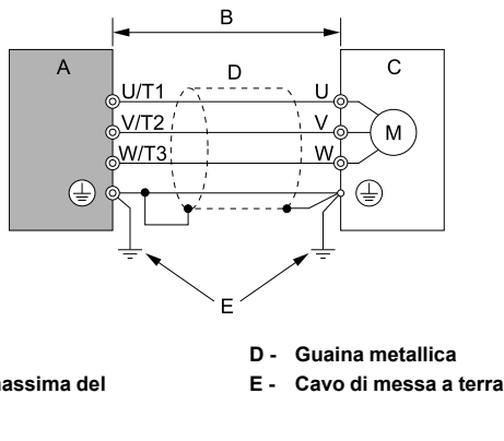
Figura 4.7 Cablare l'inverter e il motore
