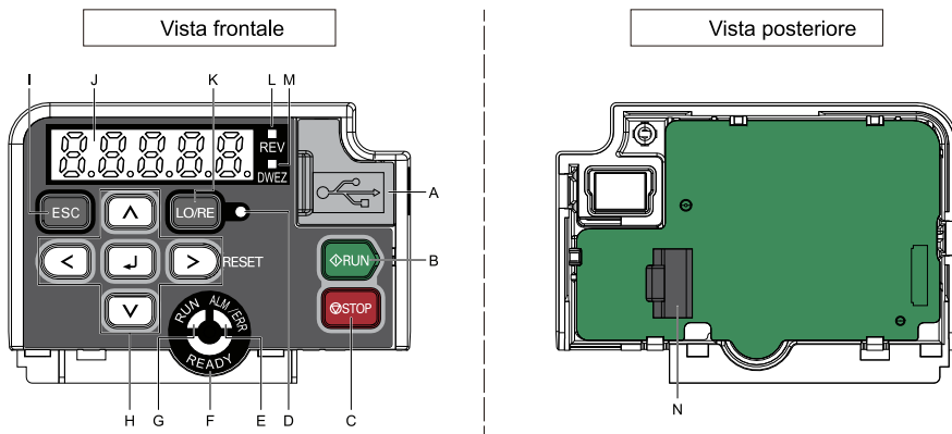
Figura 4.1 Tastiera
