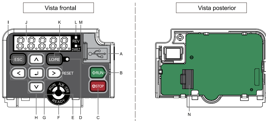
Figura 5.1 Teclado
