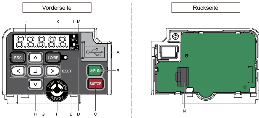
Abbildung 2.1 Bedienteil
